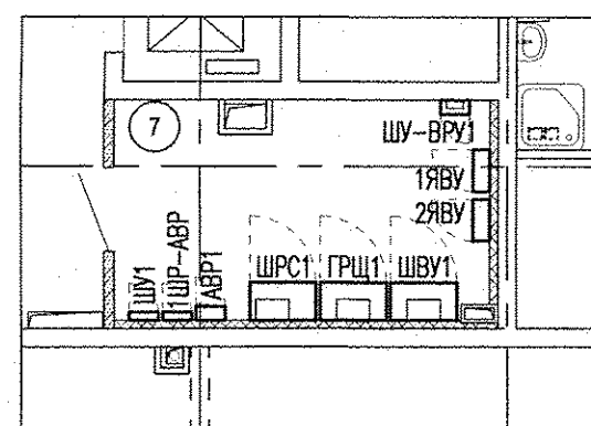
ЭЛЕКТРОЩИТОВАЯ. РАССТАНОВКА ЭЛ.ОБОРУДОВАНИЯ.
